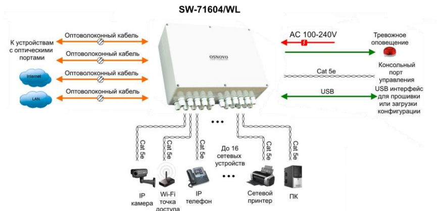
Рис.6 Типовая схема подключения коммутатора SW-71604/WL
