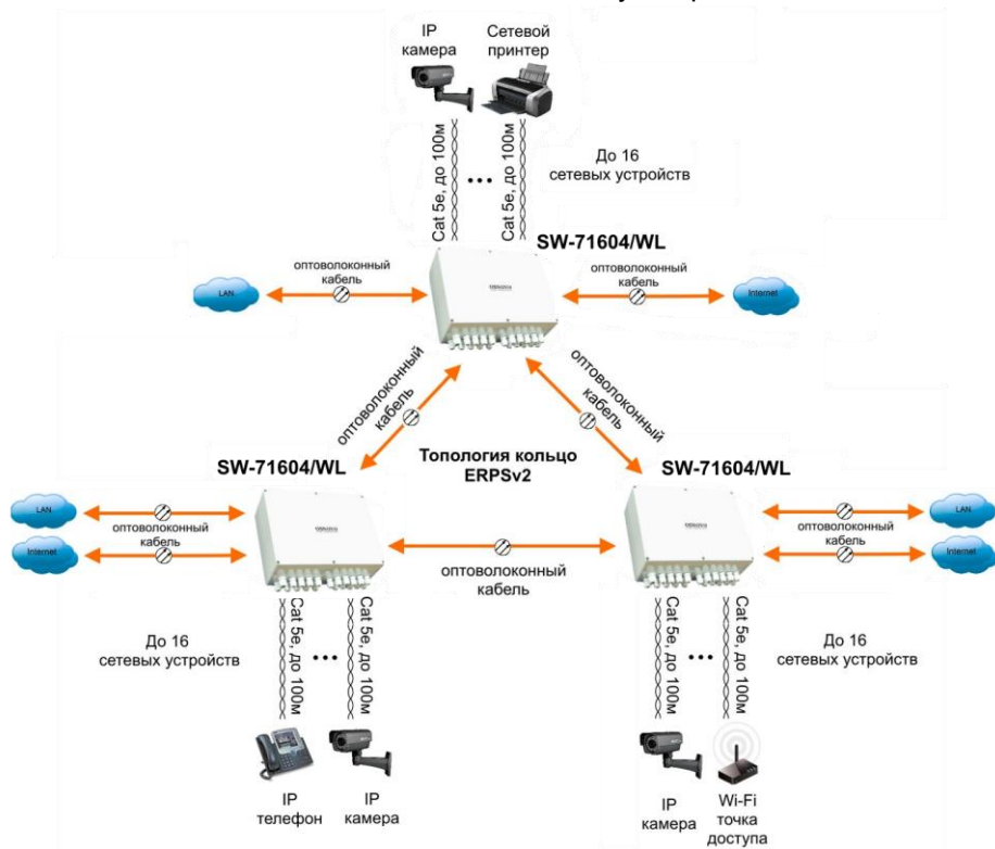
Рис.6 Типовая схема подключения коммутатора SW-71604/WL
