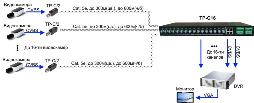
Рис.2 Схема подключения TP-C16
