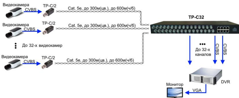
Рис.2 Схема подключения TP-C32
