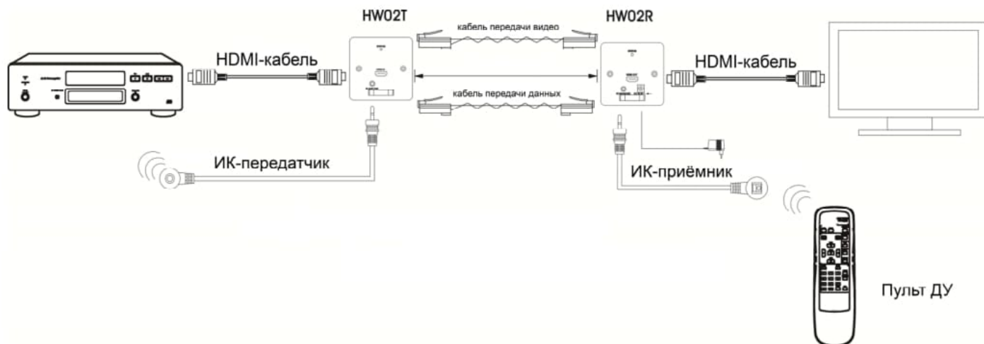
Рис. 3 Схема подключения
