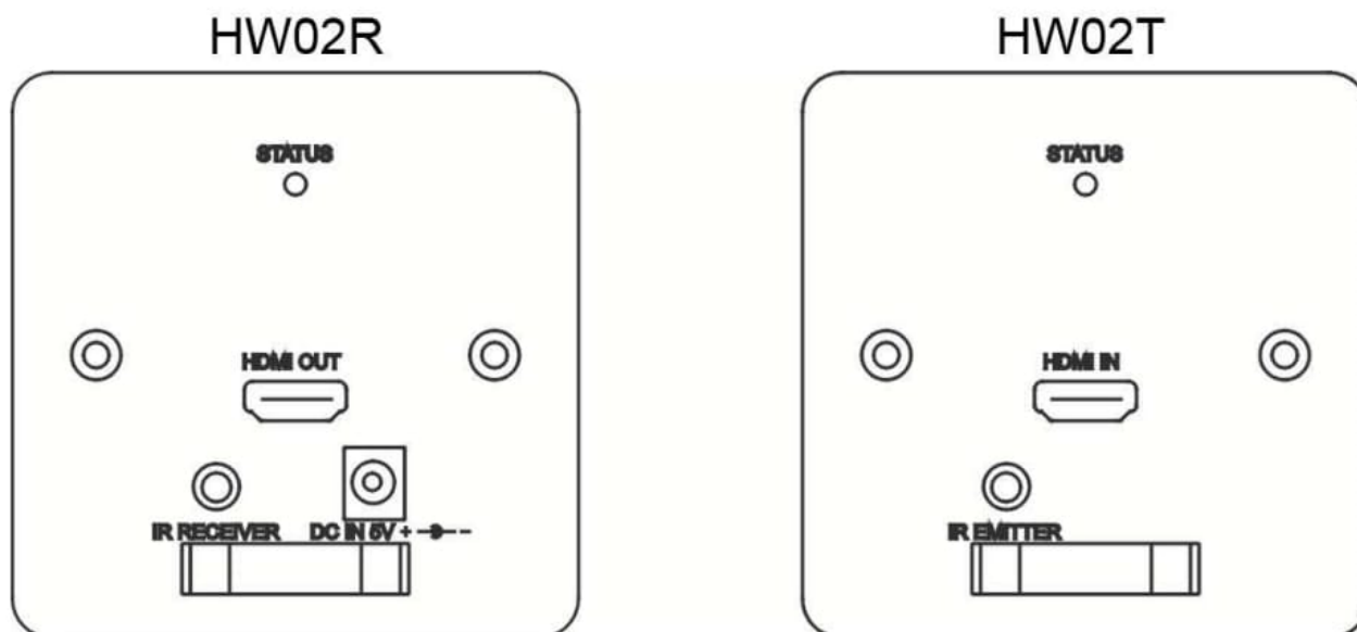
Рис. 3 Элементы HW02
