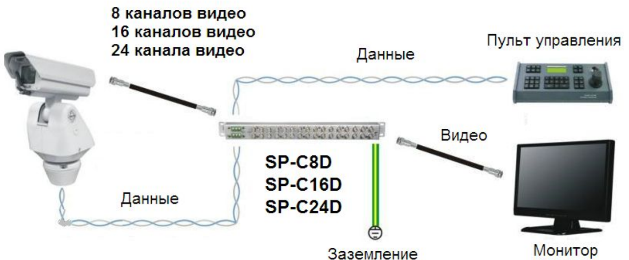
Рис.3 Подключение SP-C8D, SP-C16D, SP-C24D
