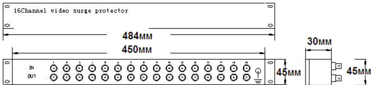
Рис.2 Габаритные размеры SP-C8D, SP-C16D, SP-C24D
