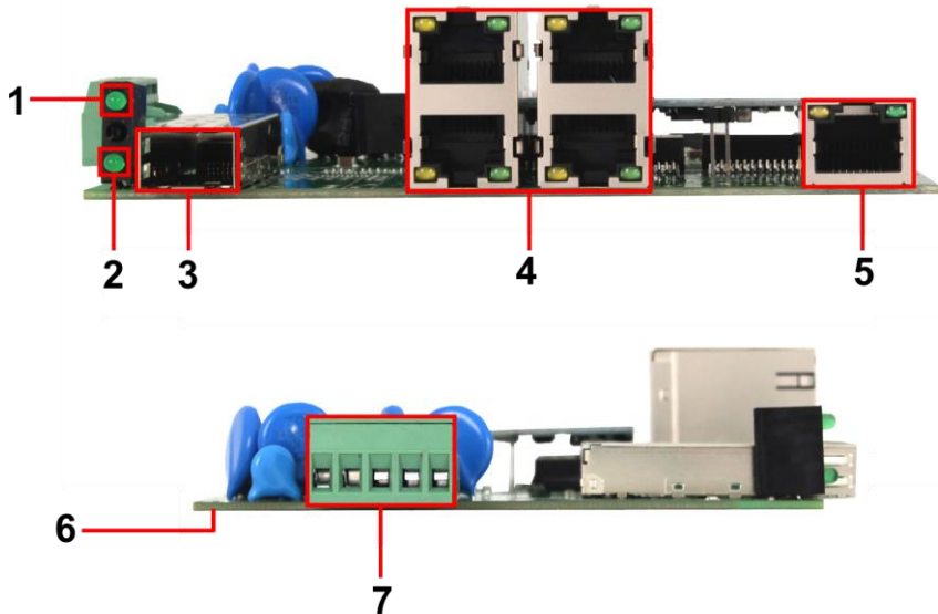
Рис. 3 Разъемы и индикаторы коммутатора SW-40501/IC-P
