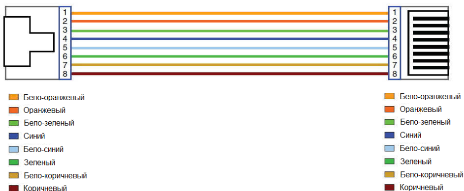
Рис. 10 Разводка кабеля по типу TIA/EIA-568-A.
