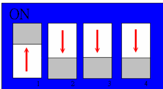
Рис. 4 Расположение DIP-переключателей на TR-IP2(CO) или TR-IP2PoE для оптимальной работы.
