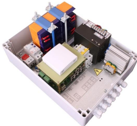
Рис.2 Уличный коммутатор SW-80802/WLU, основные элементы
