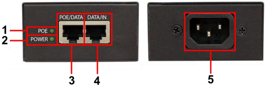
Рис. 2 Midspan-1/902G, разъемы на передней и задней панелях
