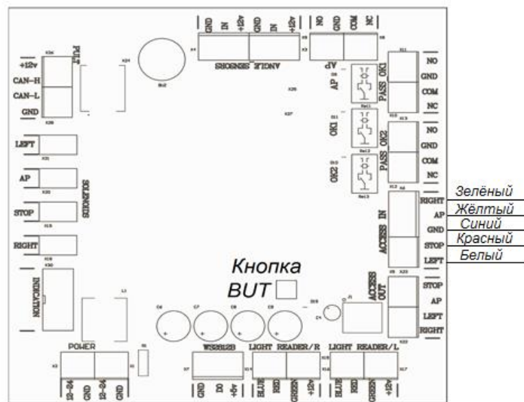
Рисунок 8.1 – Схема подключения упрощенного пульта
