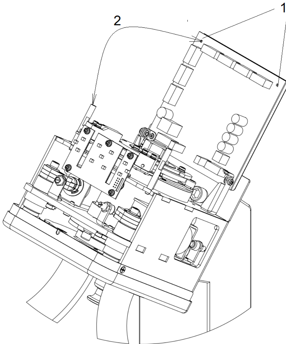
Рисунок 12 – Подключение контроллера
