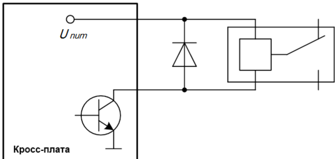
Рисунок 14 – Схема подключения диода параллельно обмотке реле
