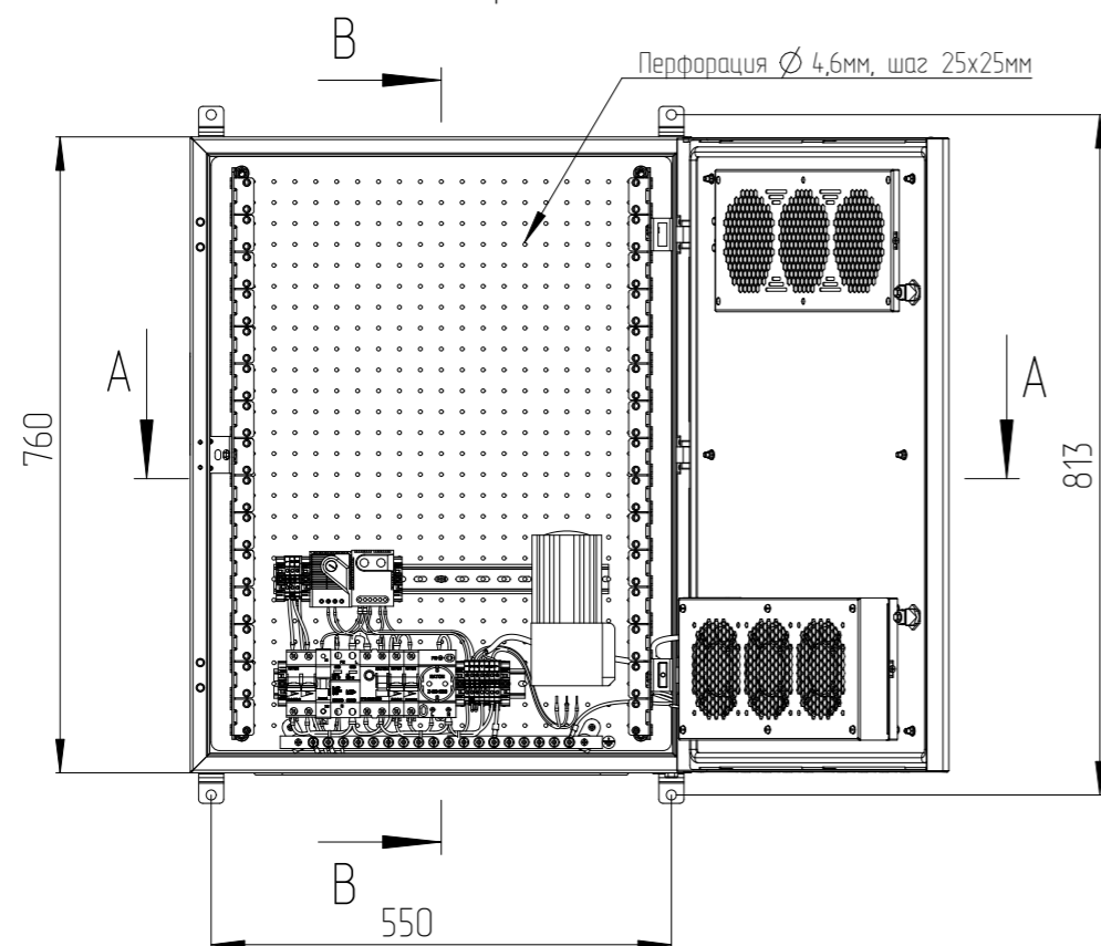
Вид спереди. Масштаб 1:10
