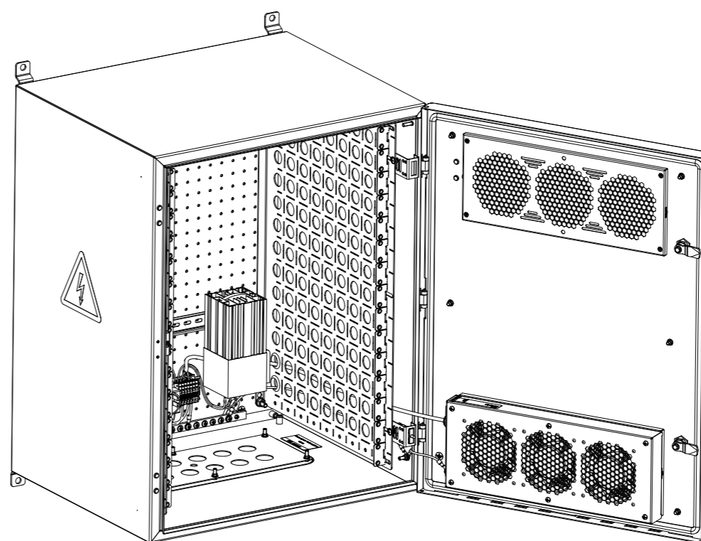
Общий вид. Масштаб 1:10
