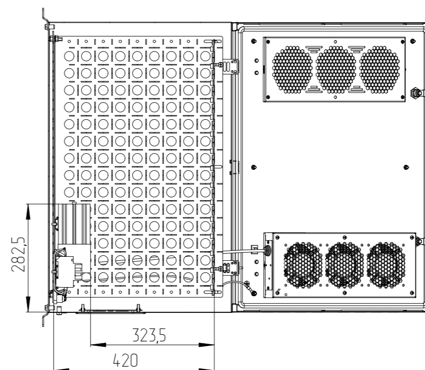
Сечение В-В. Масштаб 1:10
