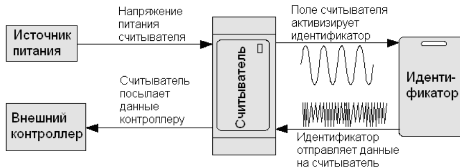
Рисунок 5. Функциональная схема, поясняющая работу считывателя
